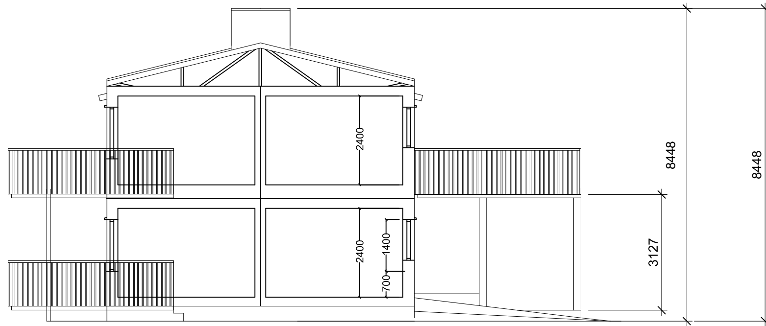
PRINCIPSEKTION
